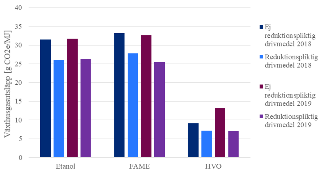
Figur 32. Genomsnittligt växthusgasutsläpp för redovisade volymer av etanol, FAME och HVO. De olika staplarna visar skillnaden mellan biodrivmedel som har ingått i ett reduktionspliktigt drivmedel respektive icke reduktionspliktigt drivmedel under 2018 och 2019.
