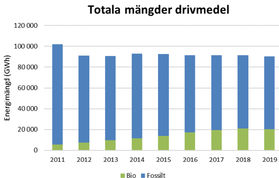
Figur 1. Totala mängden rapporterade drivmedel med innehållande mängd fossila (blått) och förnybara komponenter (grönt). Vid summering har givna konstanter enligt drivmedelslagen använts för beräkning av energimängden.
