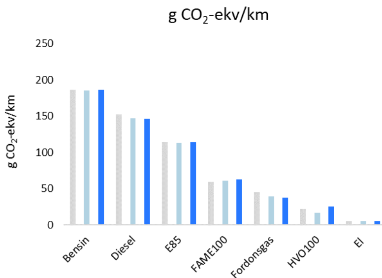
Figur 9. Växthusgasutsläpp gCO 2 ekv/km från genomsnittlig personbil med 2019 års drivmedelskvaliteter. De gråa staplarna visar 2017 och 2018 års resultat.
