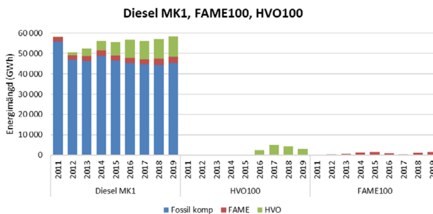
Figur 6. Leveranser av HVO och FAME inblandat i diesel MK1 och som förnybart drivmedel HVO100 och FAME100.
