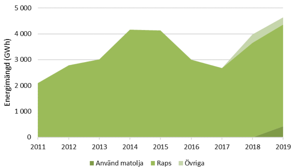
Figur 17. Råvaror till FAME 2011 till 2019, GWh.
