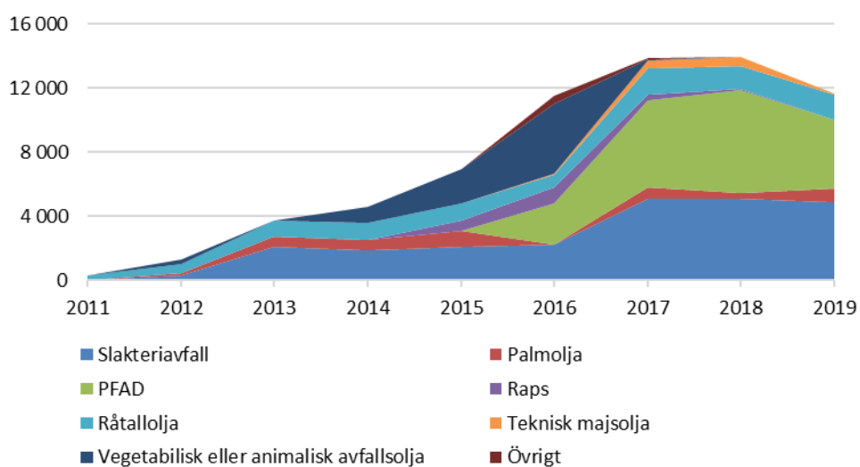
Figur 16. Utvecklingen för användning av råvaror till HVO.
